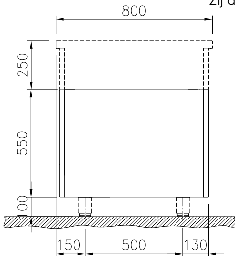
Zij aanzicht
